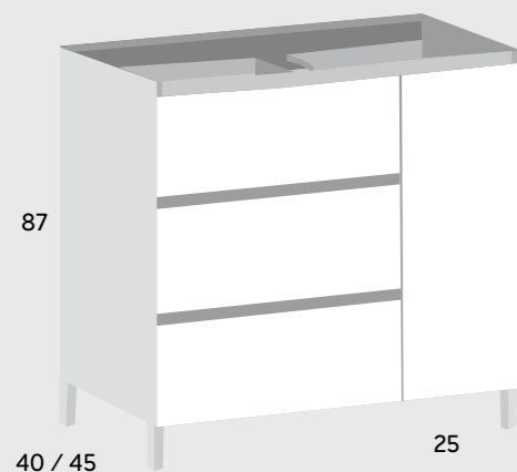
Bajo portalavabos 3 cajones, 1 puerta Bathroom unit 3 drawers, 1 door Meuble 3 tiroirs, 1 porte
